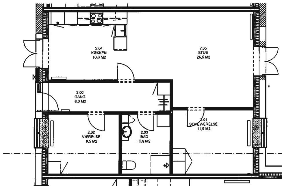
LEJLIGHED NR. 10 - 87 M 2 (TYPE 2)
